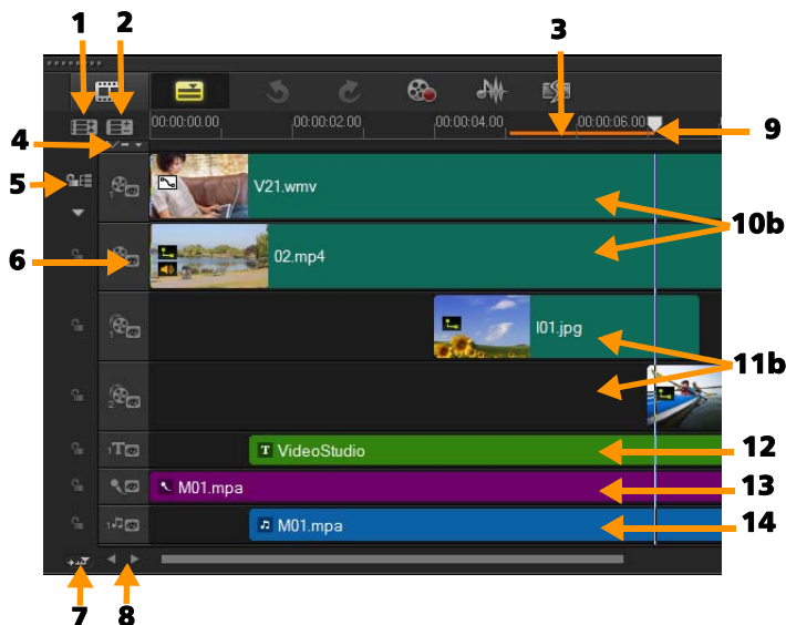
Corel VideoStudio Pro Linea temporale in modalità HTML5
