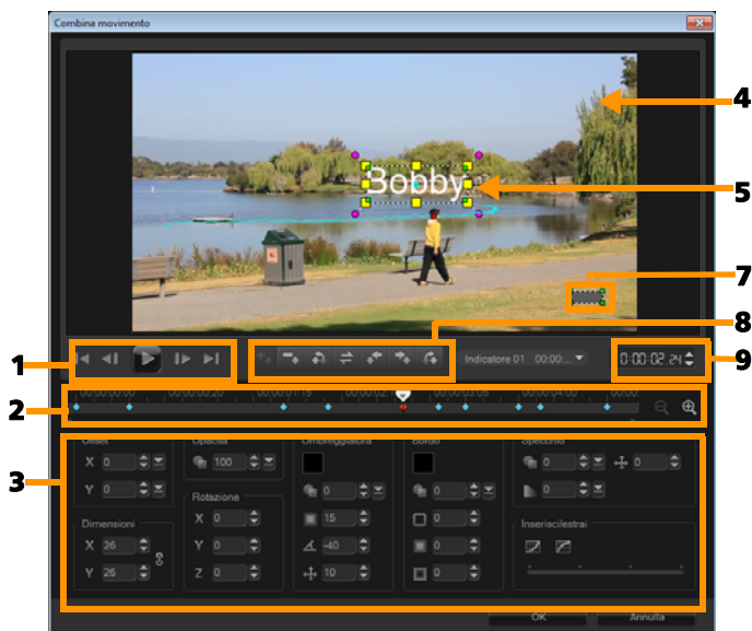
Finestra di dialogo Combina movimento
